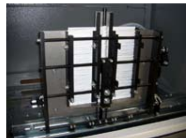
Kalenderaufhängerzuführung
