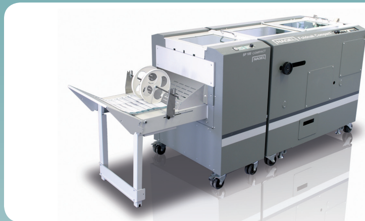
Foldnak Compact mit SP 100 Compact.
