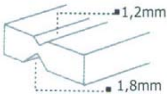
Matrize mit 2 Nuten
