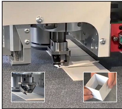
V-Schnitt für Boxen
