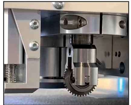
Perforierwerkzeug
