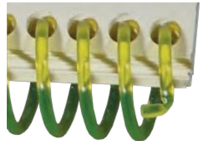
Automatisches Schneiden und 90° Crimpen
