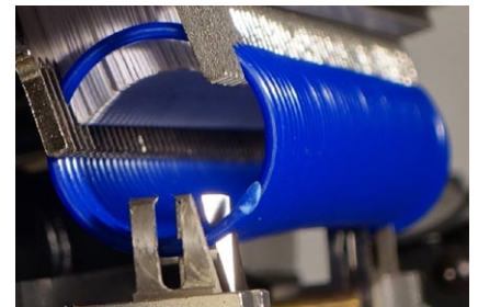
Crimpmesser und stabile Spiralführung durch Käme vorne und hinten
