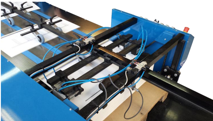
Gerader Papierlauf
