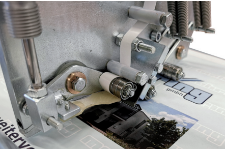
Pneumatischer Tapekopf
