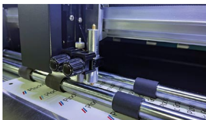
Rillen und Schneiden in einem Arbeitsgang mit Doppelwerkzeugkopf
