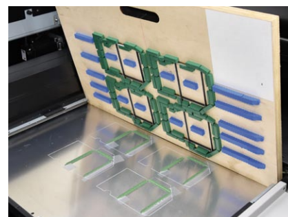
Die AeroDieCut nutzt traditionelle Bandstahlschnittwerkzeuge.
