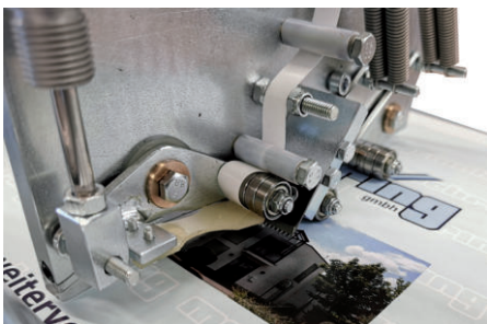
Pneumatischer Tapekopf
